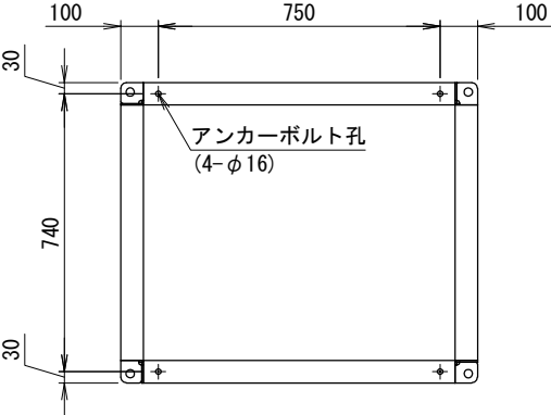
＜アンカー寸法図＞ SCALE= 1:15
