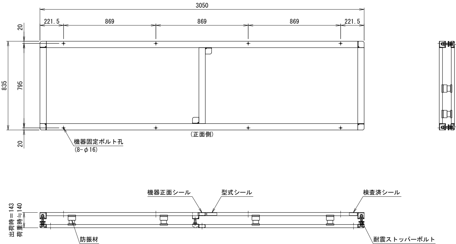
<アンカー寸法図> SCALE= 1:25
