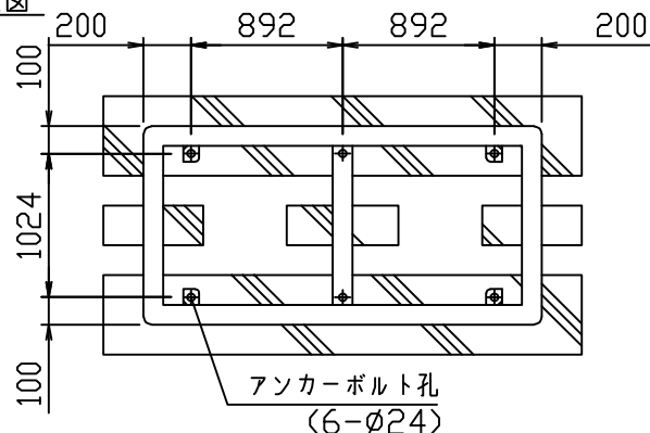
基礎図
