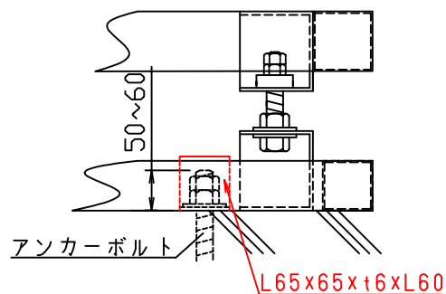
アンカー及びストッパー
