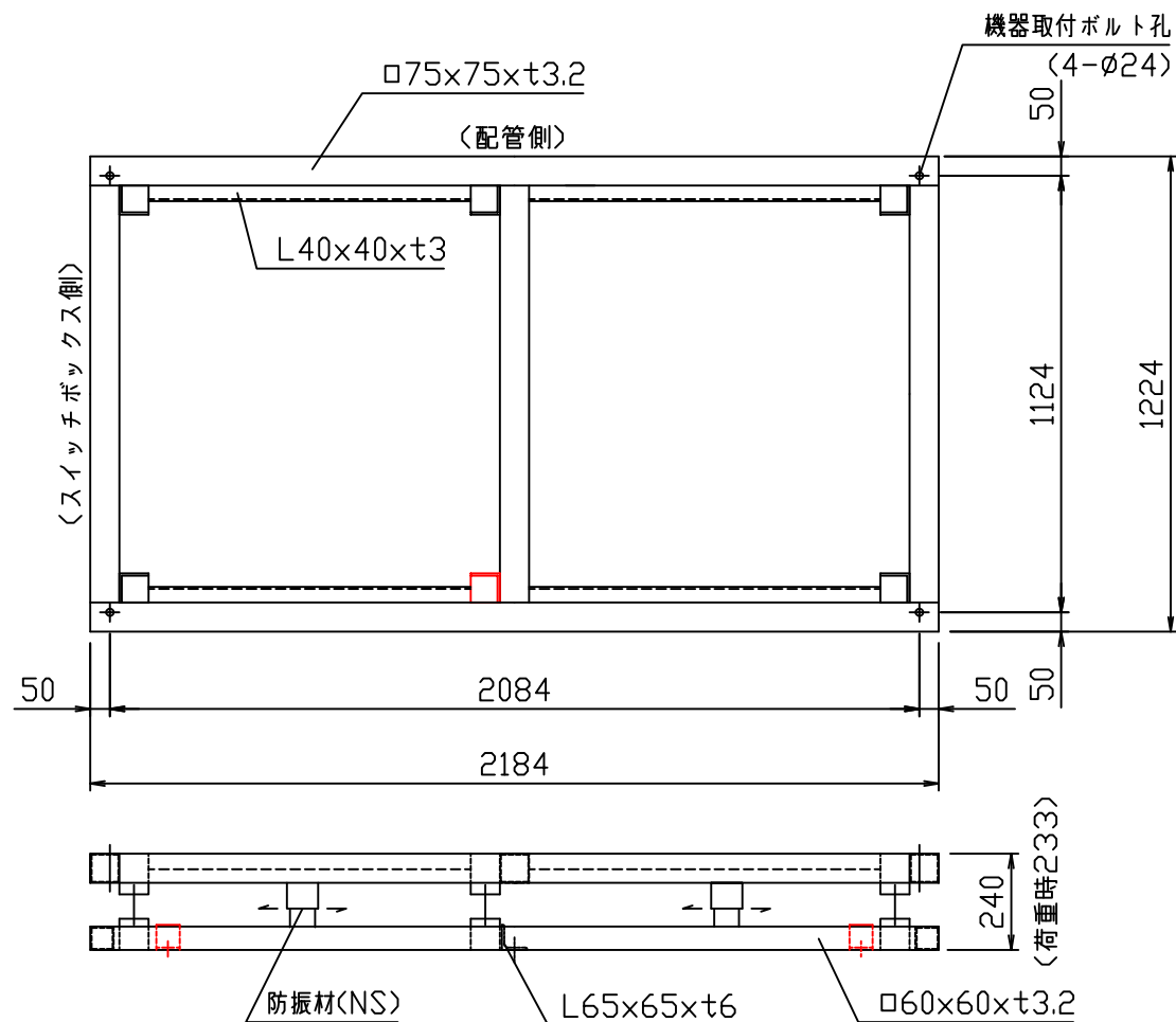
基礎図
