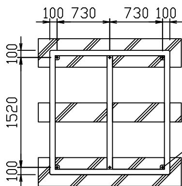
基礎図
