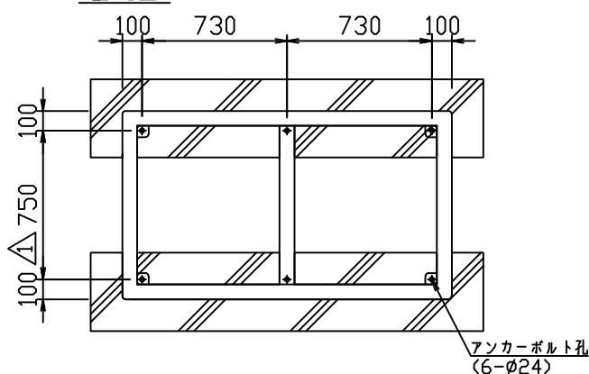
基礎図
