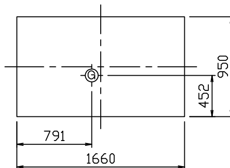
重心位置
