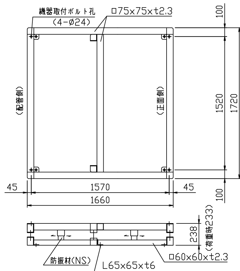
基礎図
