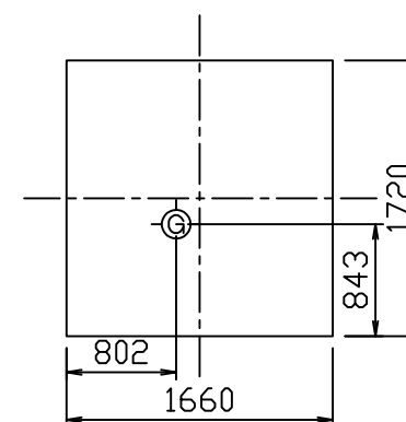
重心位置
