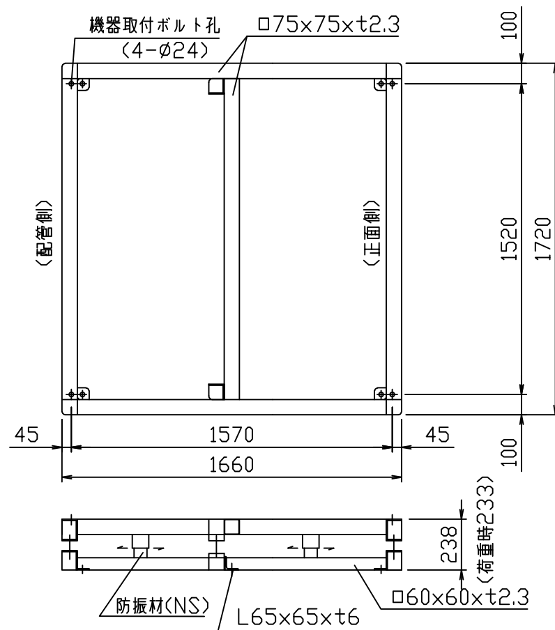
基礎図
