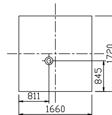
重心位置
