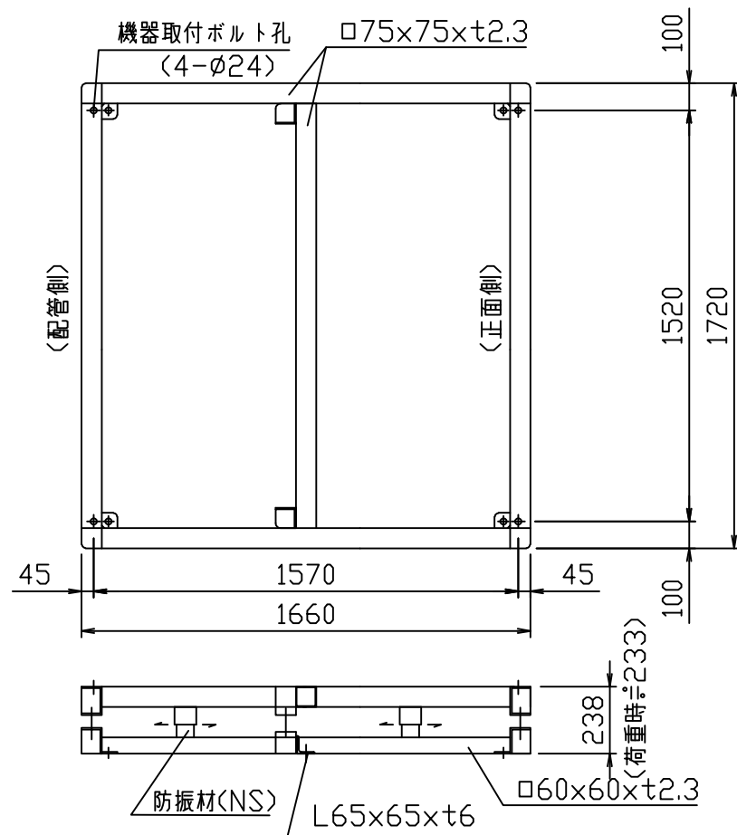
基礎図
