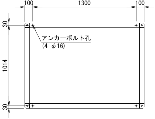
＜アンカー寸法図＞ SCALE= 1:20
