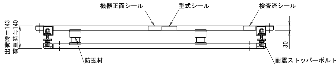
＜アンカー寸法図＞ SCALE= 1:15
