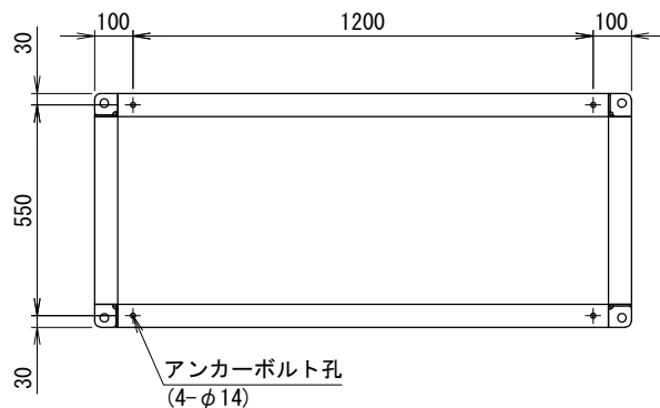
＜アンカー寸法図＞ SCALE= 1:15
