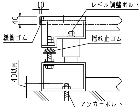
アンカー及びストッパー
