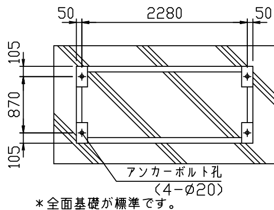
アンカー位置図
