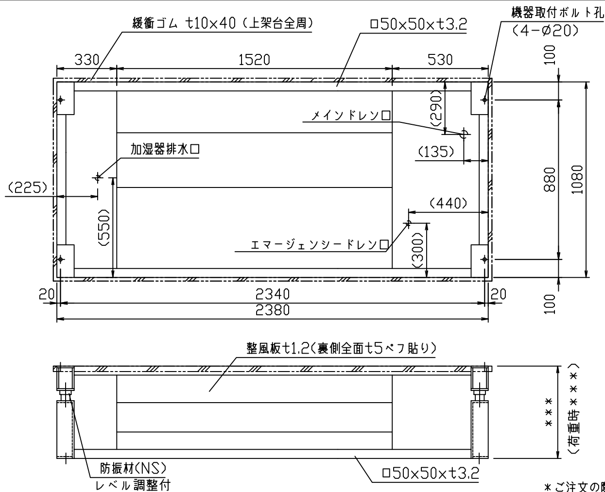
アンカー位置図
