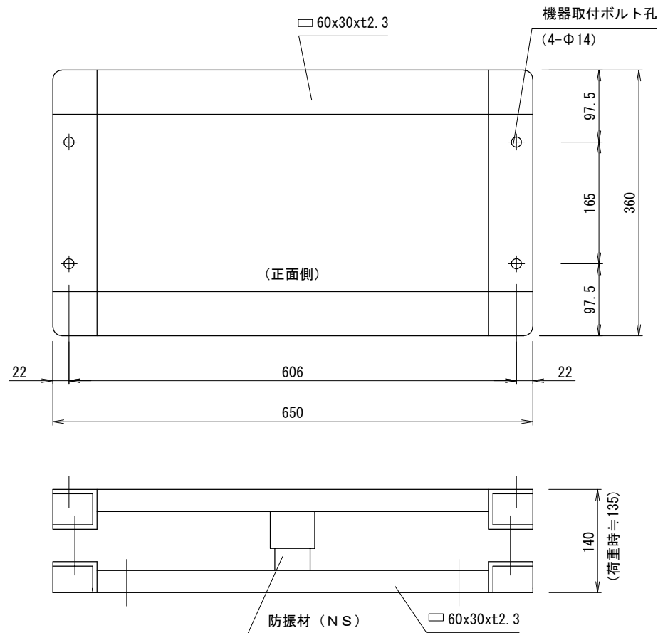
アンカー寸法図
