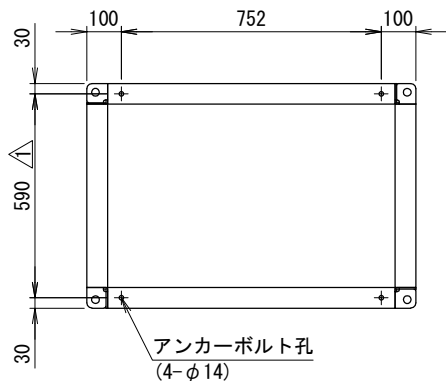
<アンカー寸法図> SCALE= 1:15
