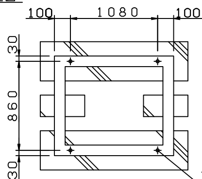
基礎図
