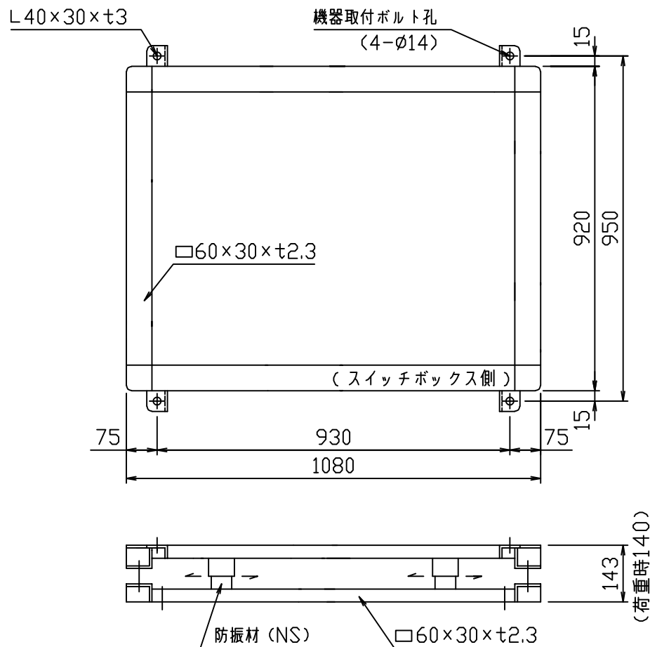
基礎図
