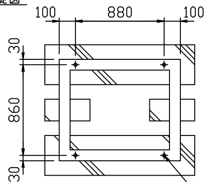
基礎図
