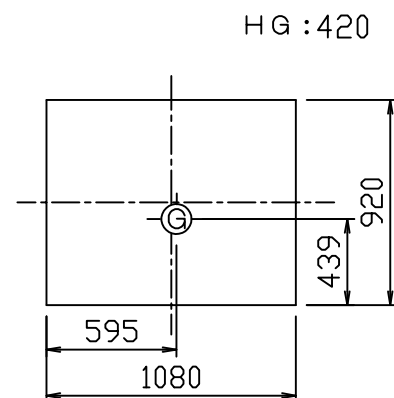
重心位置
