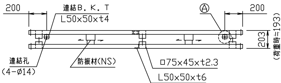
基礎図1
