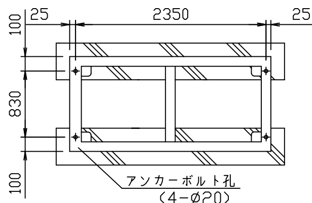
基礎図1
