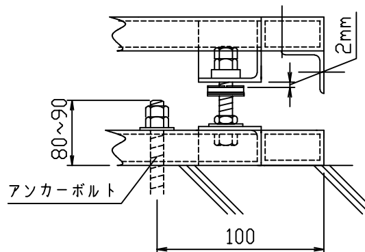
アンカー及びストッパー
