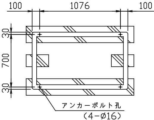
基礎図
