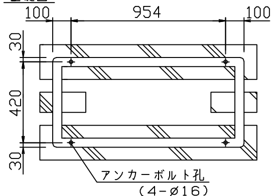
基礎図
