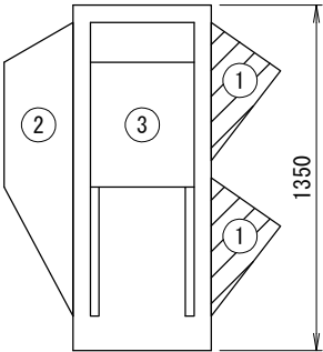
左側面図
