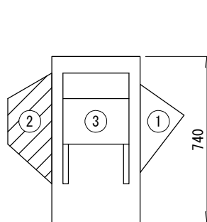
左側面図
