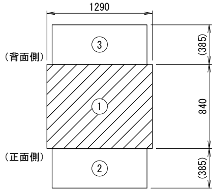
上面図
