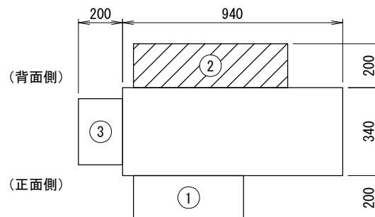
上面図
