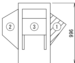
左側面図
