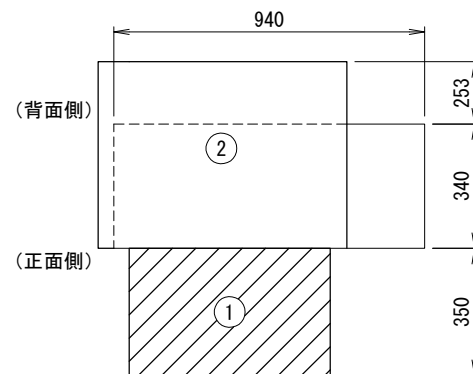
上面図
