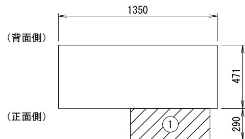
上面図
