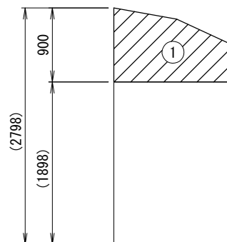
右側面図
