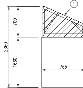
右側面図
