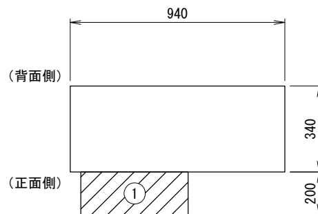
上面図
