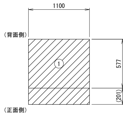
上面図
