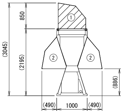
正面図
