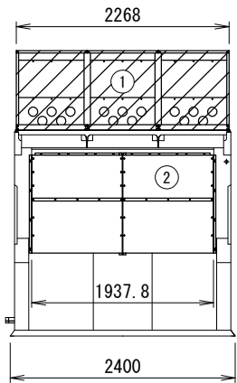
左側面図
