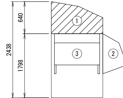
右側面図
