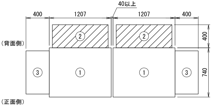
上面図
