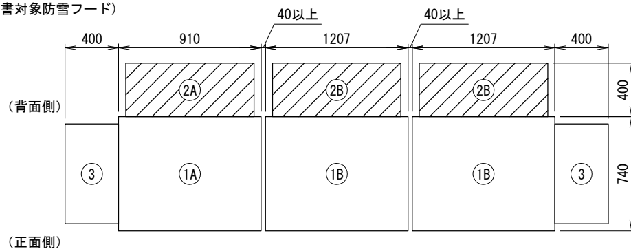
上面図
