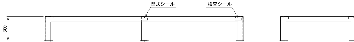
<アンカー寸法図> SCALE= 1:20
