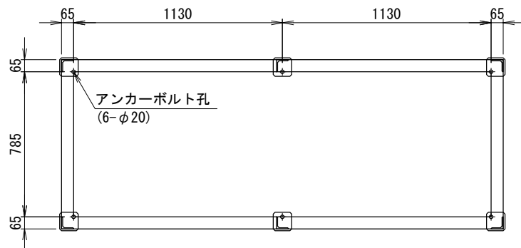
<アンカー寸法図> SCALE= 1:20
