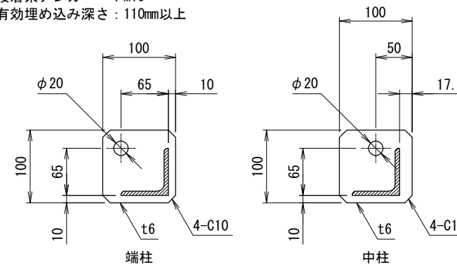
<アンカー部詳細>(対称形状)
