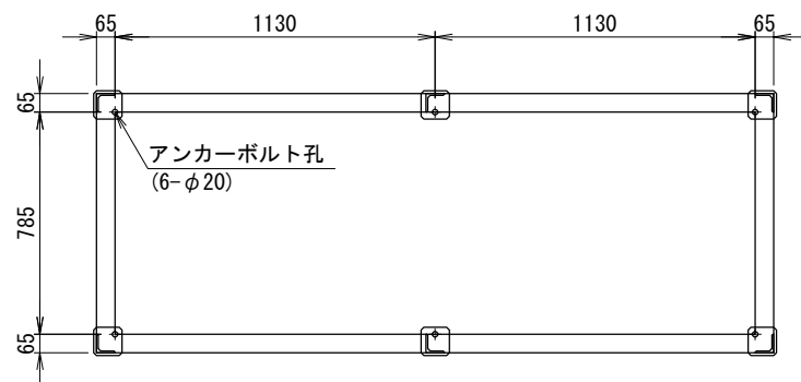
<アンカー寸法図> SCALE= 1:20
