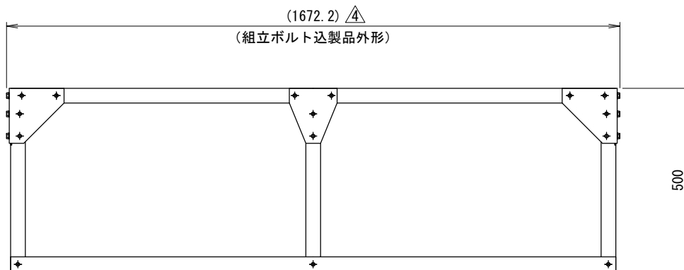
取付棧 (SUS304)
