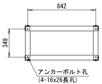
<アンカー寸法図(長孔中心)> SCALE= 1:20 アンカー金具取付(A)内側
