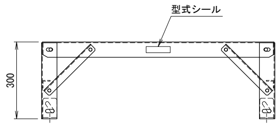
アンカー金具取付(B)外側側面
