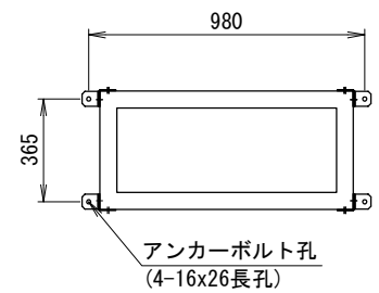
アンカー金具取付(B)外側側面
