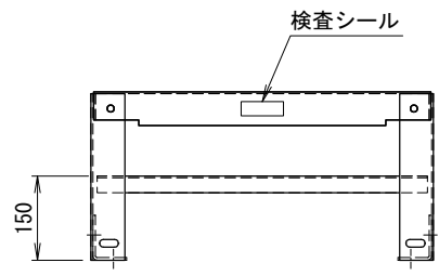
アンカー金具取付(C)外側前後面
