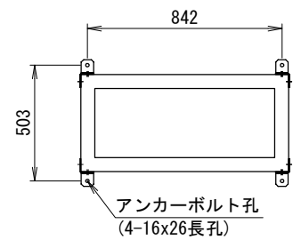
アンカー金具取付(C)外側前後面
