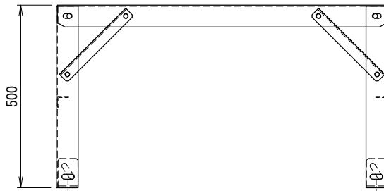
アンカー金具取付(B)外側側面
