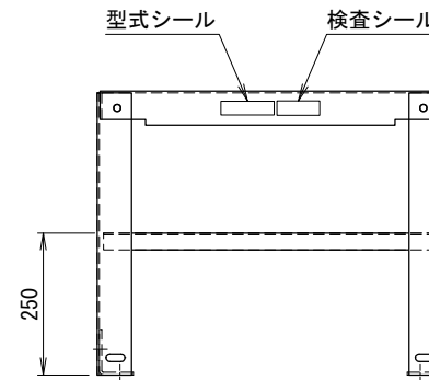
アンカー金具取付(C)外側前後面
