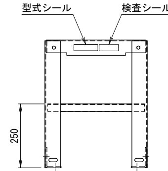
アンカー金具取付(C)外側前後面
