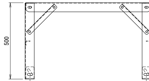
アンカー金具取付(B)外側側面
