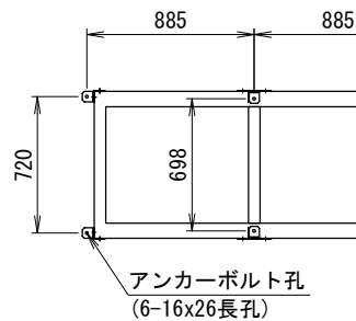
アンカー金具取付(B)外側側面
