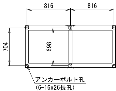
<アンカー寸法図(長孔中心)> SCALE= 1:30 アンカー金具取付(A)内側
