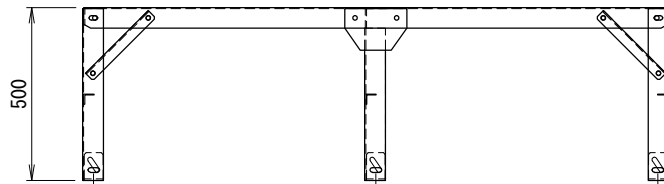
<アンカー寸法図(長孔中心)> SCALE= 1:30 アンカー金具取付(A)内側
