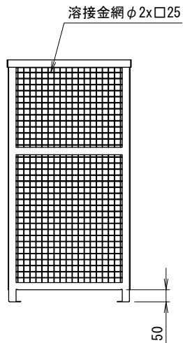
左側面図
