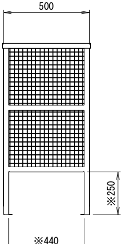
右側面図
