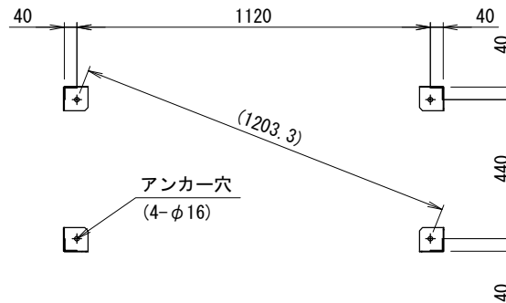
アンカー寸法図
