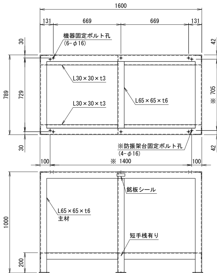
〈アンカー寸法図〉 SCALE= 1:15
