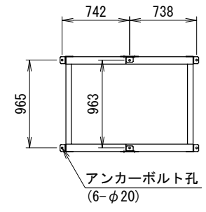
アンカー金具取付 (B)
