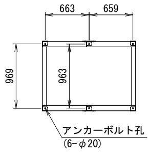
<アンカー寸法図> SCALE= 1:40 アンカー金具取付 (A)
