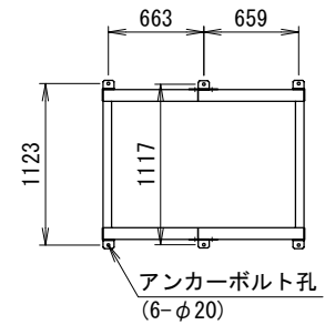
アンカー金具取付 (C)
