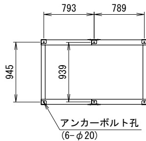
<アンカー寸法図> SCALE= 1:40 アンカー金具取付 (A)
