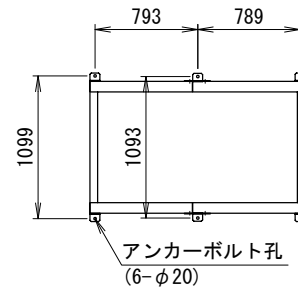
アンカー金具取付 (C)
