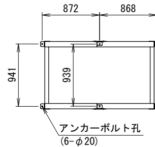
アンカー金具取付 (B)
