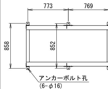
アンカー金具取付 (C)
