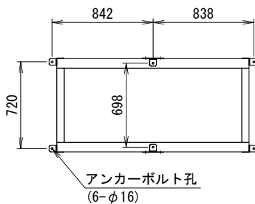
アンカー金具取付 (B)
