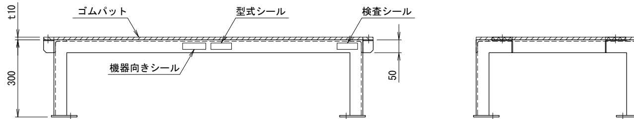
<アンカー寸法図> SCALE= 1:12
