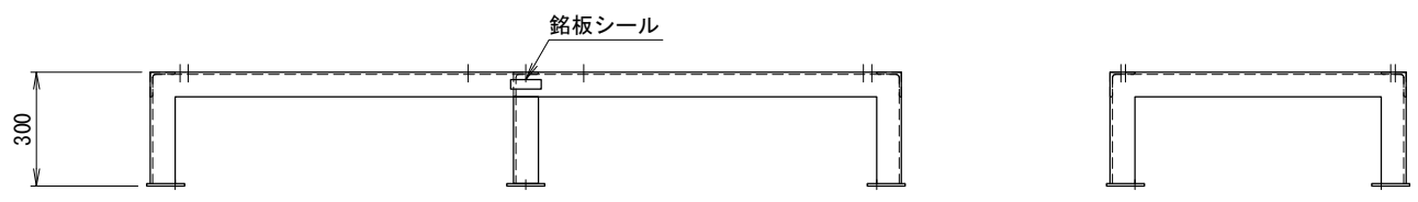
<アンカー寸法図> SCALE= 1:15
