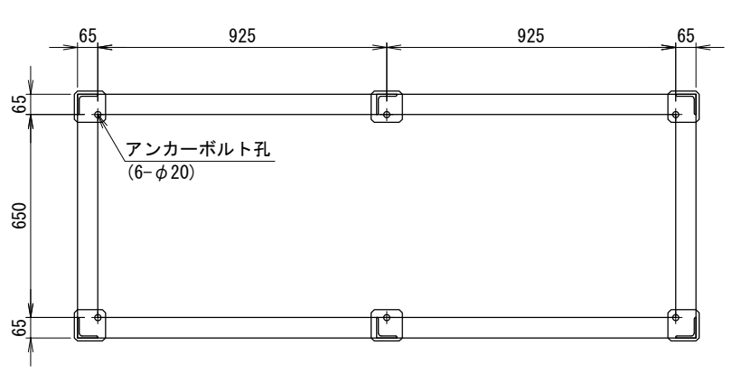
<アンカー寸法図> SCALE= 1:15
